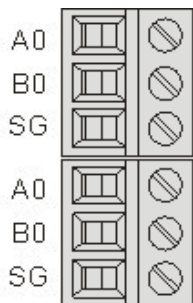
2 группы 3-х контактных клемм, расположенных на расстоянии 3.81 мм друг от друга
