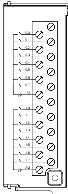
SM3DI16
