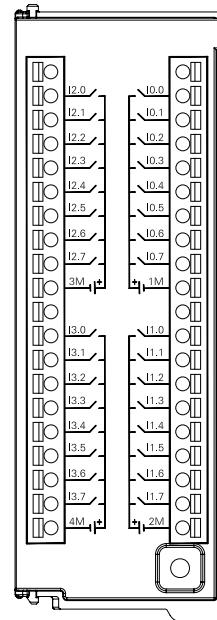
SM3DI32
