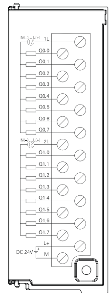
SM3DQ16R
