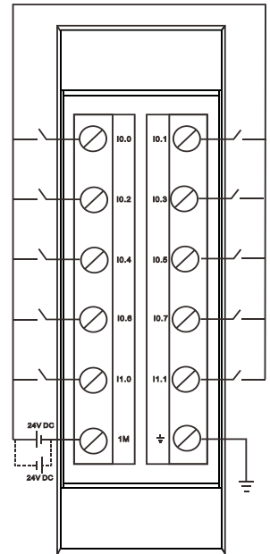
Дискретные входы контроллера SM253CE10
